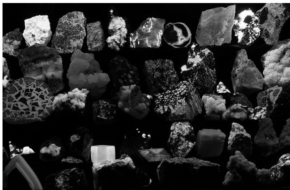
Exemple de roches fluorescentes
